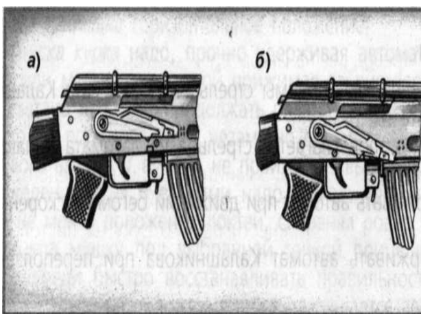
Рис. 6 Установка переводчика на необходимый вид огня: а - для ведения автоматического огня; б - для ведения одиночного огня
